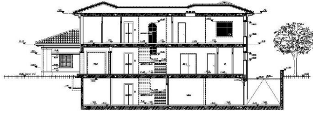
F - F KESİTİ
