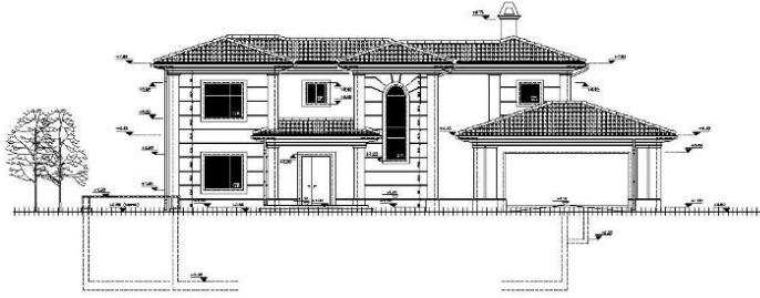
ÖN CEPHE
