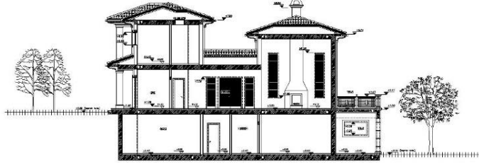
E-E KESİTİ
