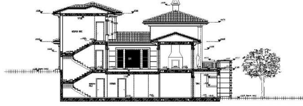
A - A KESİTİ
