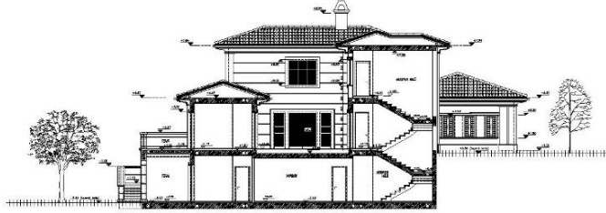
C - C KESİTİ
